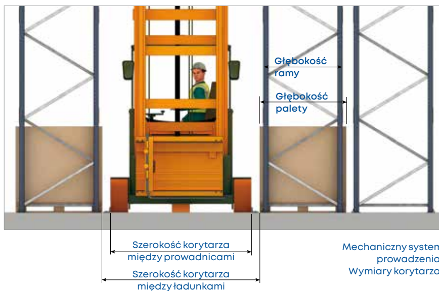
Schemat mechanicznego systemu prowadzenia.
