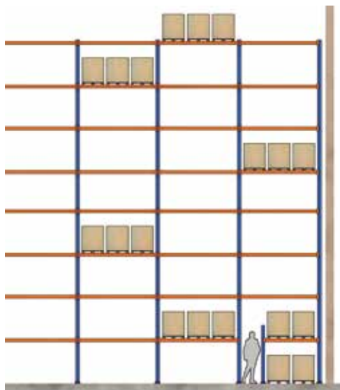
Instalacja z przejściem poprzecznym – widok z boku
